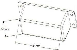
Cutout Dimensions
