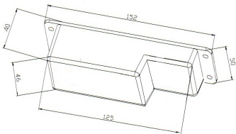
Cutout Dimensions
