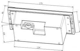
Cutout Dimensions
