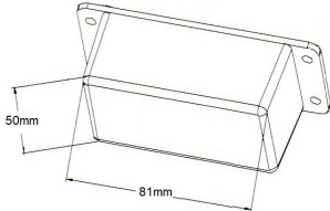
Cutout Dimensions
