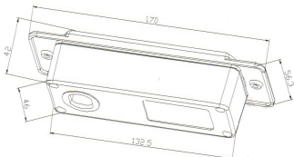
Cutout Dimensions
