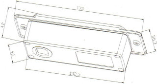
Cutout Dimensions
